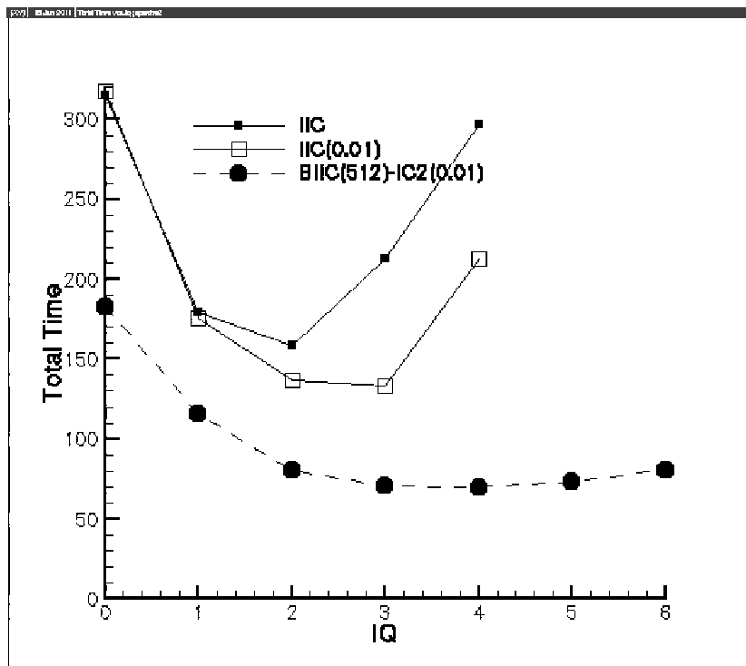
Фиг.4. Общее время счета м.с.г. в зависимости от степени перекрытия q для методов IC(q) , IC(q;0.01) и BIIC(512;q)-IC2(0.01) и задачи apache2 .
