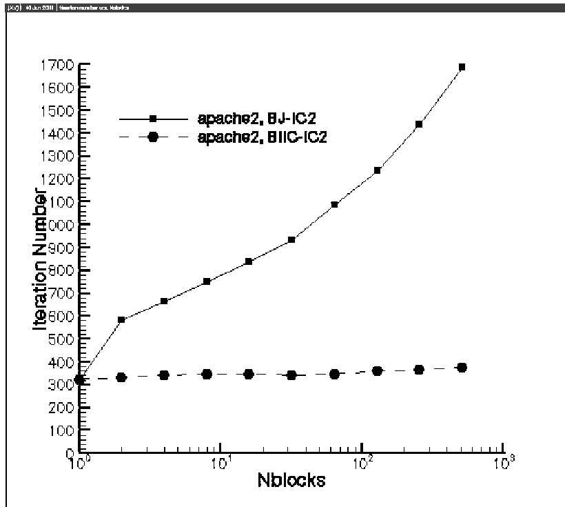
Фиг.1. Число итераций м.с.г. в зависимости от числа блоков для предобусловливания VJ(p) -IC2(0.01) и BIC(p;4) -IC2(0.01) и задачи apache2 .
