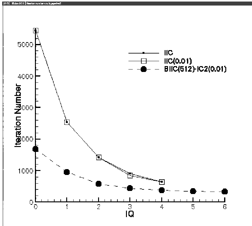
Фиг.3. Число итераций м.с.г. в зависимости от степени перекрытия q для методов IC(q) , IC(q;0.01) и BIIC(512;q)-IC2(0.01) и задачи apache2 .
