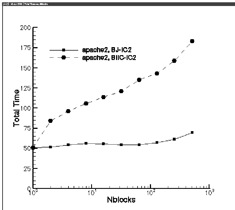
Фиг.2. Общее время счета м.с.г. в зависимости от числа блоков p для предобусловливания VJ(p) -IC2(0.01) и BIC(p;4) -IC2(0.01) и задачи apache2 .
